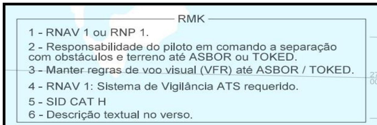
Figura 06 – Exemplo de RMK de SID PinS
